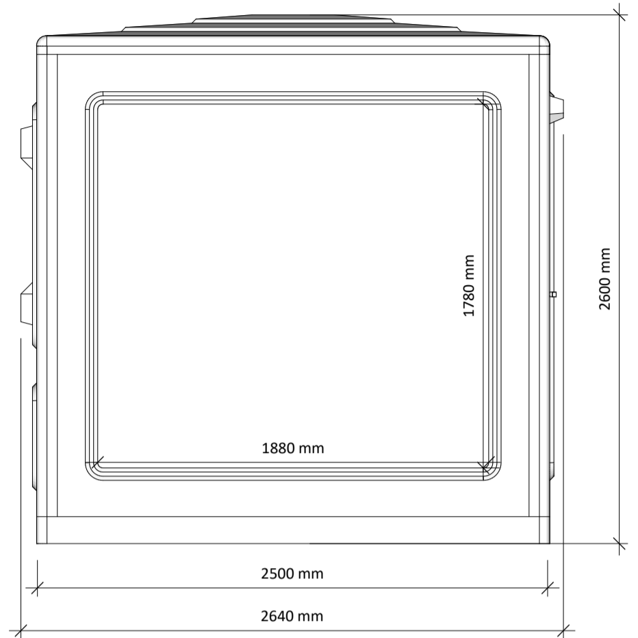
ELEVATION 'B'
