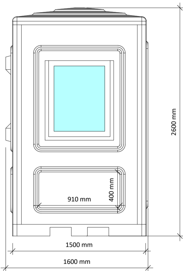
ELEVATION 'C'
