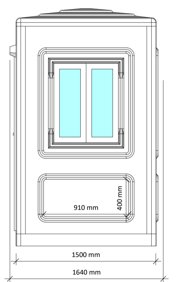
ELEVATION 'D'
