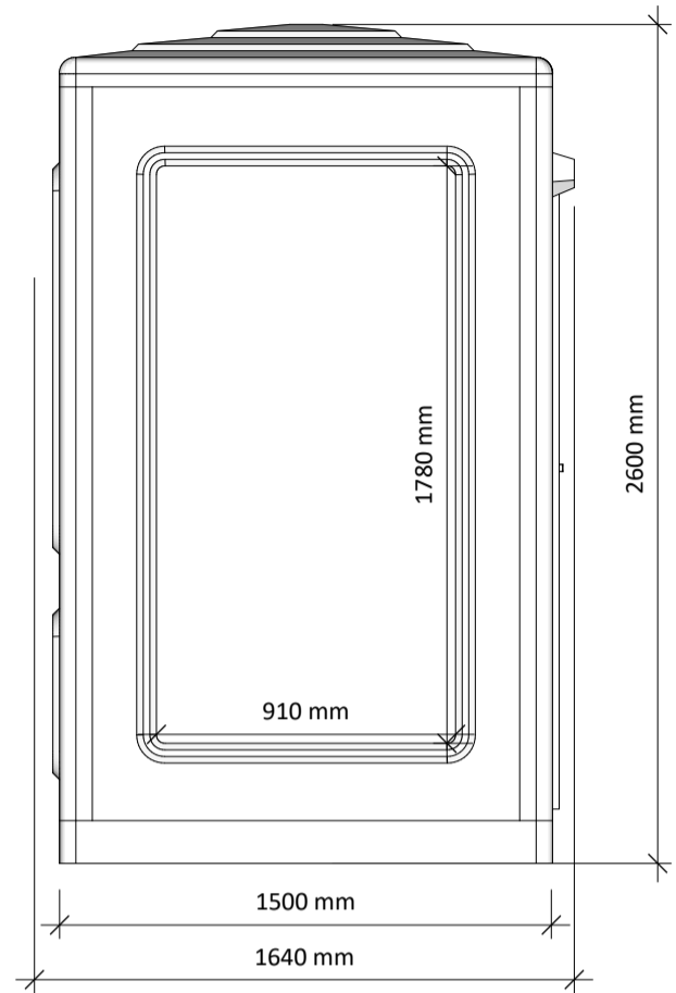
ELEVATION 'B'
